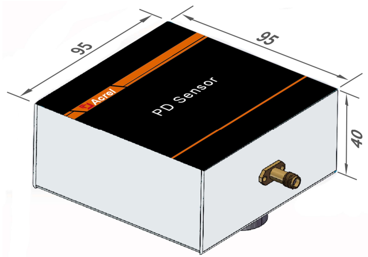
图 1.3 特高频局放传感器
