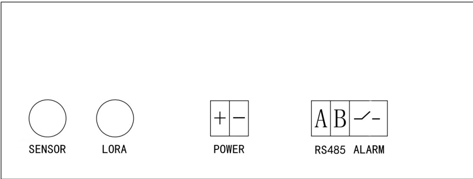
图 1.4 APD100 端子图
