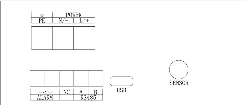
图 1.5 APD200 端子图
